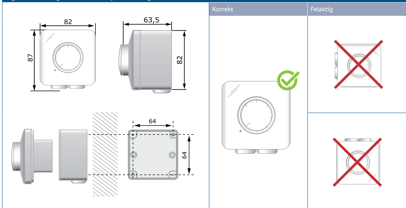
Fig. 3 Monteringsdimensioner - ytmontering
